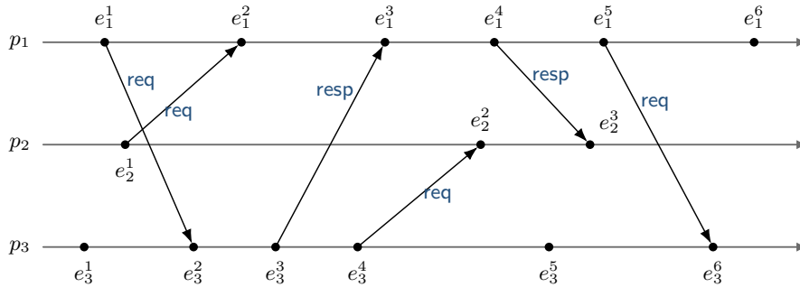
Figura 1.2. La computazione d'esempio: tre processi che si scambiano richieste (req) e risposte (resp).
