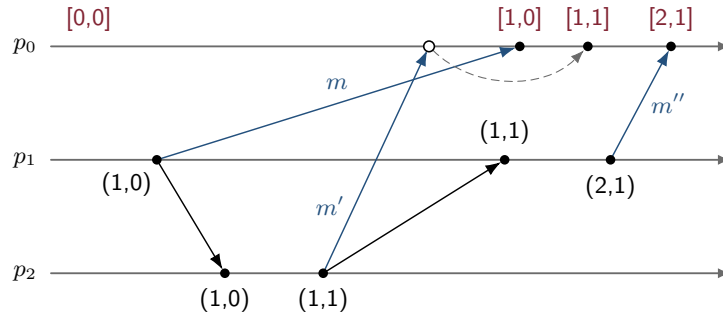
Figura 4.4. La regola DR3 al lavoro. Su p_1 e p_2 i vector clock, su p_0 (in rosso) i valori di D ; in blu le notifiche. m' arriva prima di m (cerchio vuoto) e viene consegnata solo dopo di essa.
