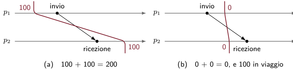
Figura 1.1. Il bonifico dell'esempio: il tempo scorre da sinistra a destra, e la freccia è il messaggio con i 100 euro. Le linee rosse passano per i punti in cui le richieste di p_0 arrivano a p_1 e a p_2 ; accanto, in rosso, i saldi comunicati.
