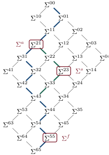
Figura 5.2. Lo snapshot nel reticolo della Figura 2.3. Il run reale (blu) passa per l'avvio \Sigma^a = \Sigma^{21} e la fine \Sigma^f = \Sigma^{55} , ma non per lo stato costruito \Sigma^s = \Sigma^{23} . Il run riordinato (verde) se ne discosta solo tra \Sigma^{21} e \Sigma^{43} , e passa per tutti e tre.
