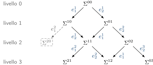
Figura 2.4. I primi livelli del reticolo della Figura 2.3, con l'evento eseguito a ogni passo. Da \Sigma^{10} non si può eseguire e_1^2 , che riceve un messaggio non ancora inviato: \Sigma^{20} non è consistente.
