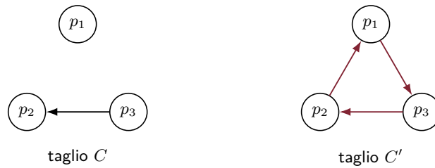
Figura 2.2. Il grafo delle attese costruito sullo stato del taglio C e su quello di C' : solo il secondo contiene un ciclo.
